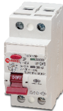
2 Kutuplu, 300 mA
