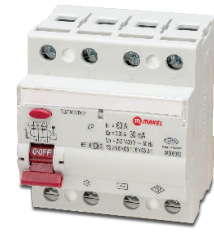
4 Kutuplu, 30 mA
