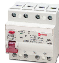
4 Kutuplu, 300 mA
