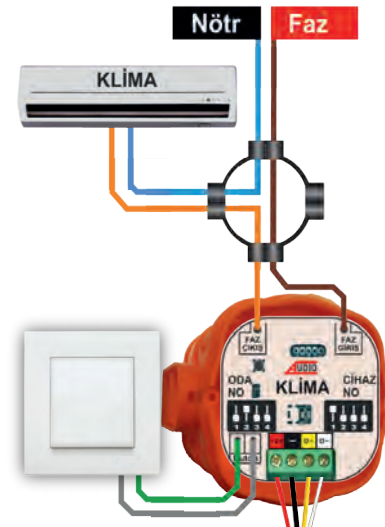
KLİMA BAĞLANTISI
