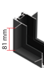
90° Dikey Bağlantı Aparatı Sıvaaltı 90° Vertical Joint Recessed
